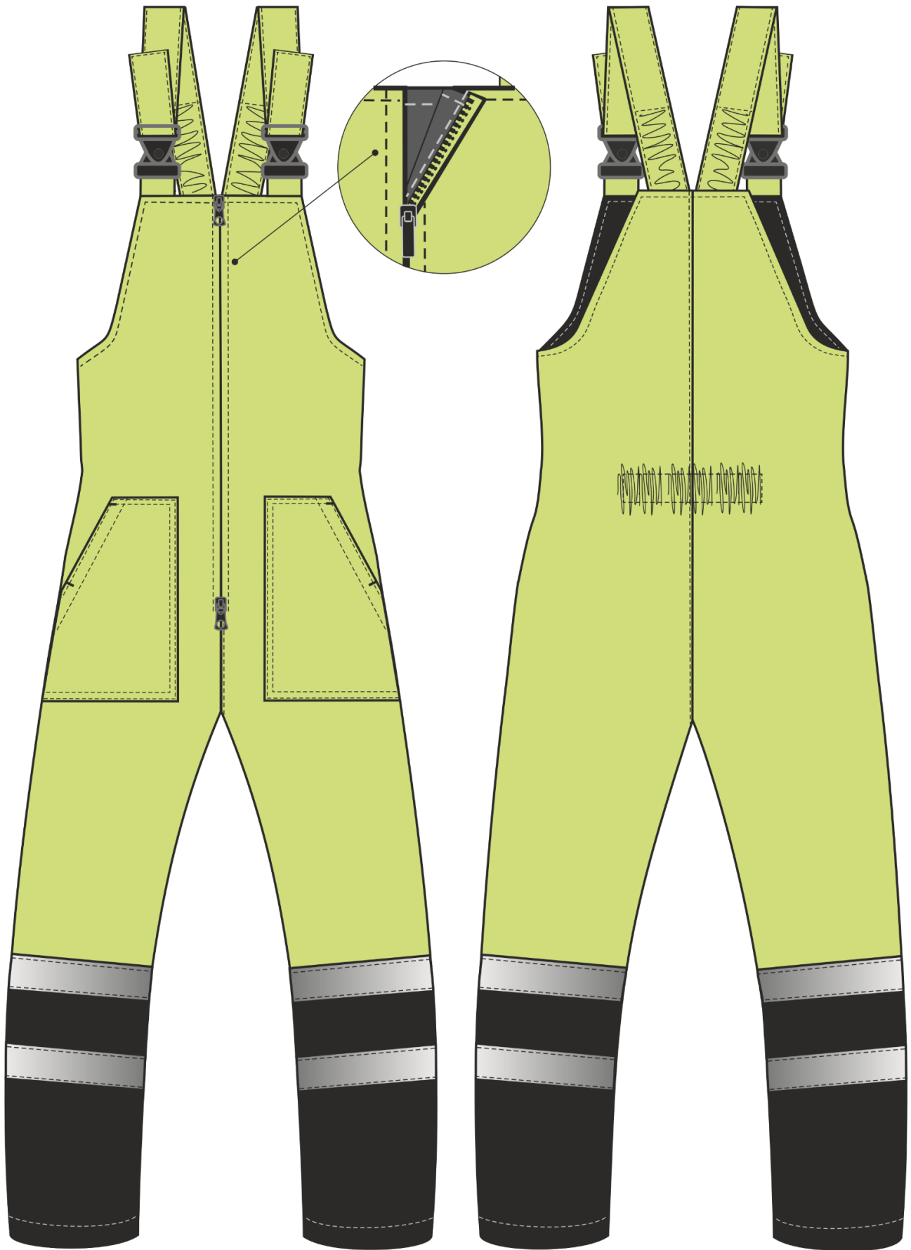
Рис.4. Эскиз Костюм зимний Дорожник-Ультра (тк.Смесовая,210) п/к, лимонный/черный. Полукомбинезон, вид спереди и сзади.
