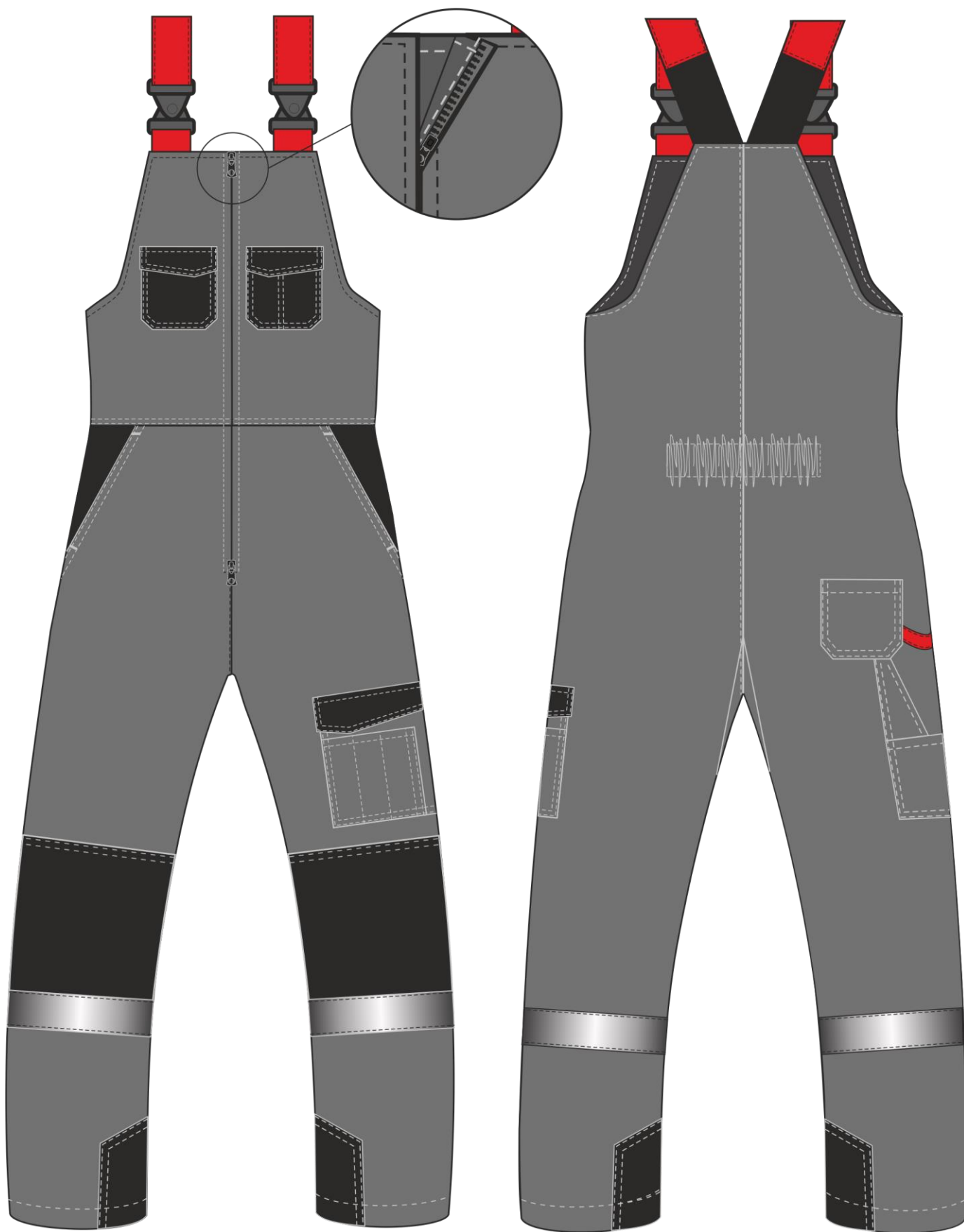
Рис. 4. Эскиз Костюм зимний Фаворит-Мега UZ (тк.Смесовая,240) п/к, серый/черный/красный. Полукомбинезон, вид спереди и сзади.
