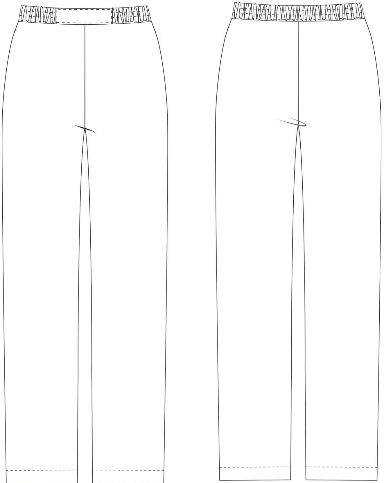
Рис. 1. Эскиз Брюки женские ХАССП-Премиум. Вид спереди и сзади.
